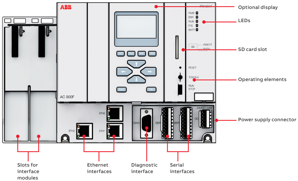
03 CPU module PM 901F
